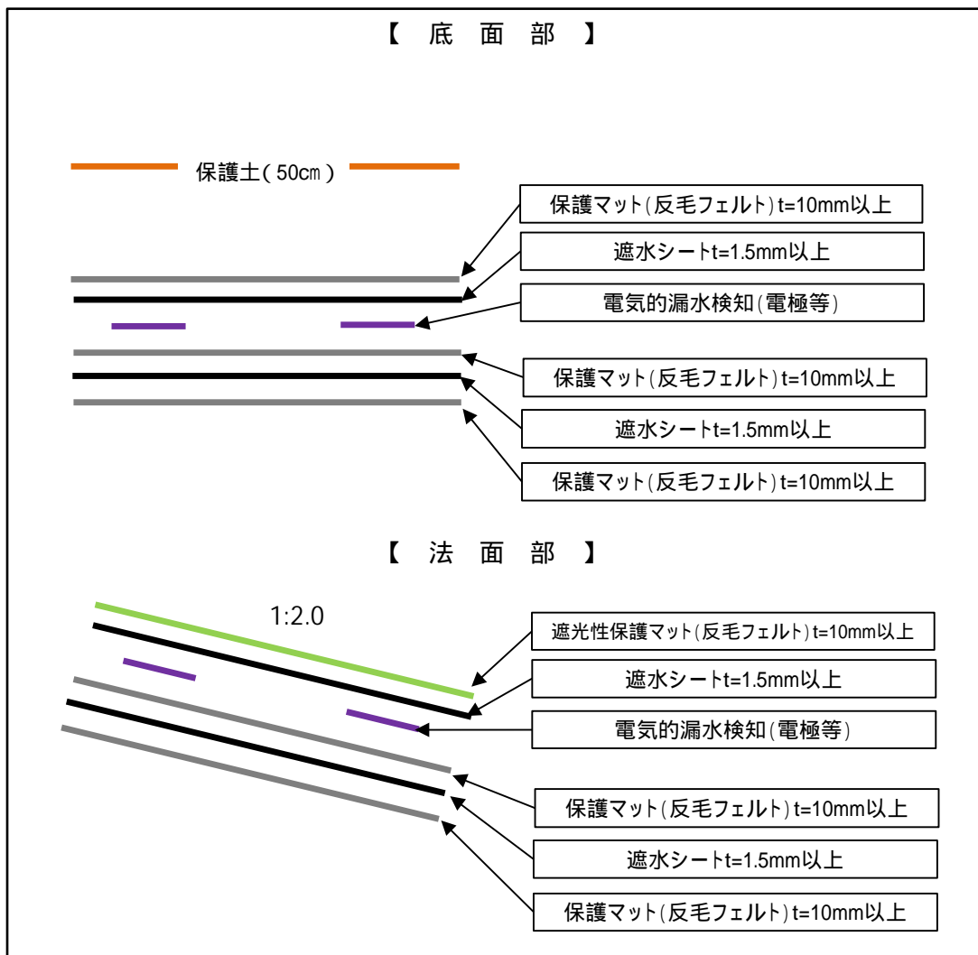
図 6.5-19 地下水浸透防止対策
