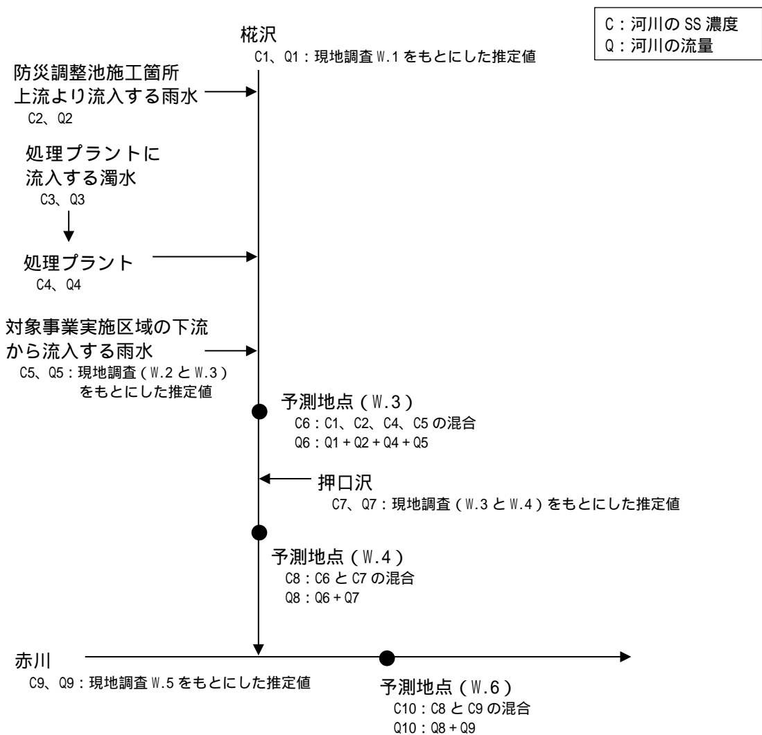
図 6.5-8 予測モデル（ 期整備時：防災調整池整備前）
