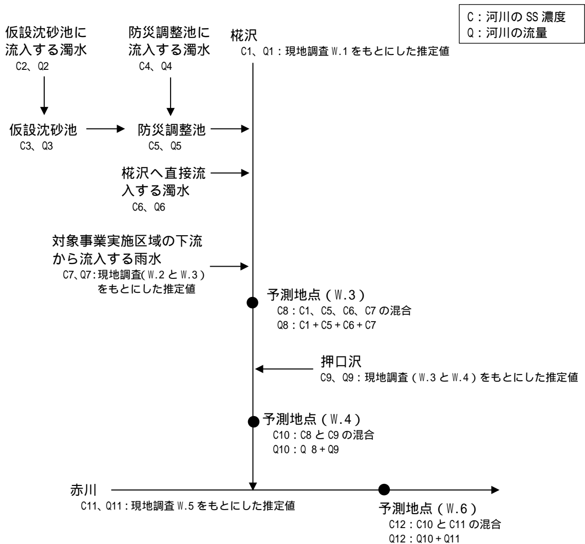
図 6.5-10 予測モデル（ 期整備時：防災調整池整備後）
