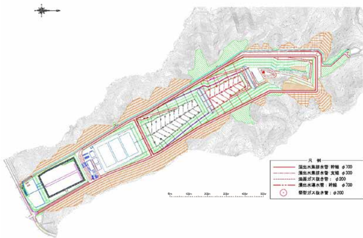
図 2-8 浸出水集排水設備の配置（Ⅱ期整備時）
